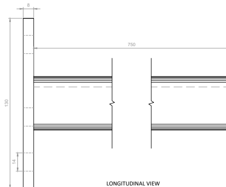
LONGITUDINAL VIEW
