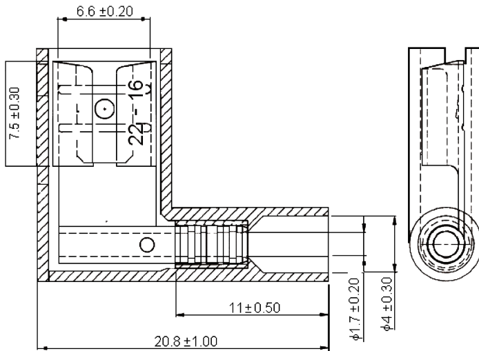
Dimensions : Millimetres
