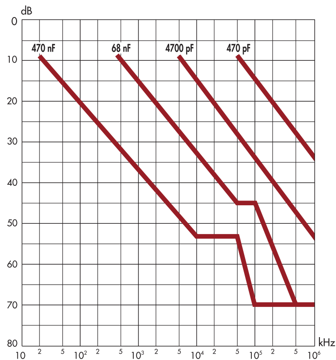
Atténuation sur 50 \Omega (à vide)
