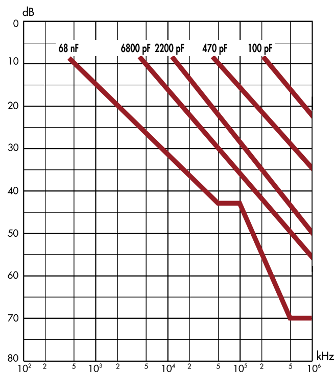
Atténuation sur 50 \Omega (à vide)
