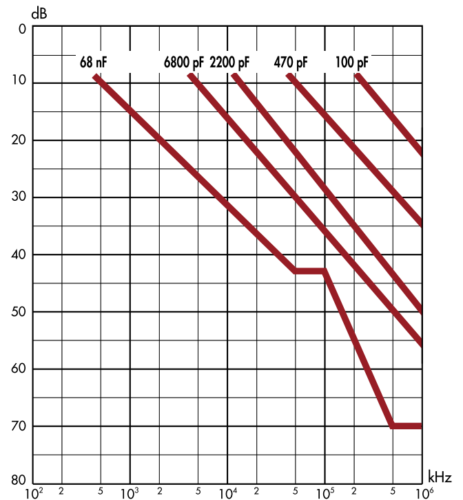
Atténuation sur 50 \Omega (à vide)
