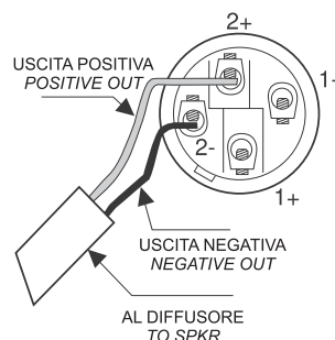
CONNESSIONE DI USCITA BRIDGE BRIDGE OUT CONNECTION
