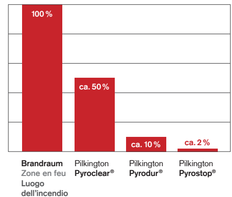
Energiedurchgang bei unterschiedlichen Brandschutzverglasungen nach 30 Minuten Normbrand / Transmission d'énergie des différents vitrages de protection incendie après 30 minutes d'exposition au feu normalisé / Passaggio di energia in varie vetrature resistenti al fuoco dopo 30 minuti di incendio standard
