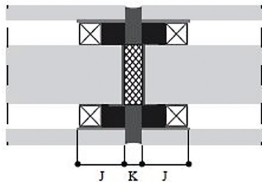
Horizontalschnitt Stossfuge
