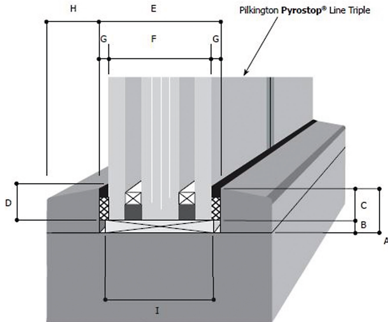
Horizontalschnitt Stossfuge
