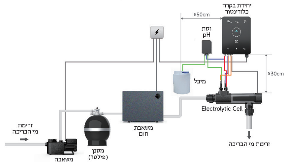
1. תרשים התקנה
