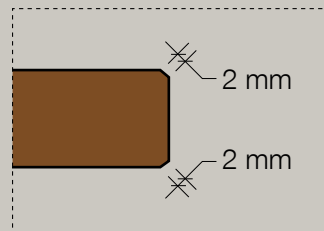
Costa Retta | Straight Edge Chant Droit | Gerade Kante
