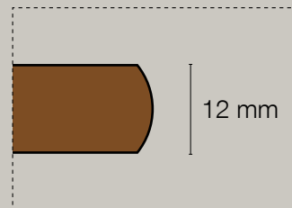
Costa a Toro | Bullnose edge Chant arrondi | Gerundete Kante r=11 mm
