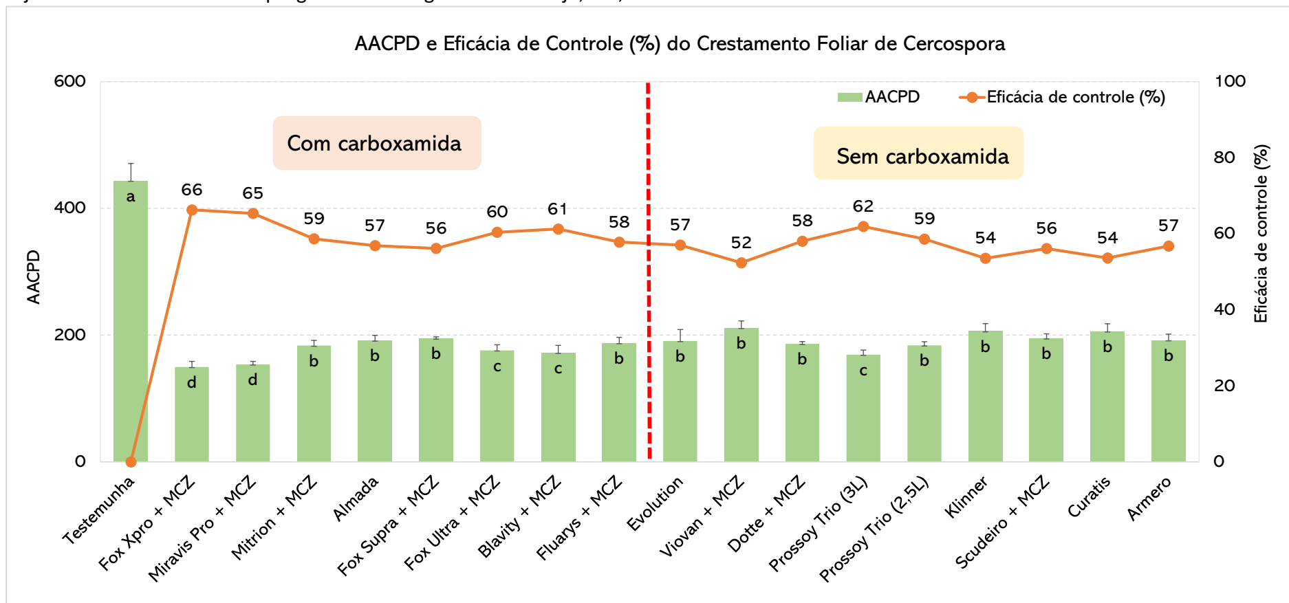
Figura 3. Área Abaixo da Curva de Progresso da Doença (AACPD) e eficácia de controle (%) do crestamento foliar de cercospora em plantas de soja submetidas a diferentes programas de fungicidas. Maracaju, MS, 2026.
