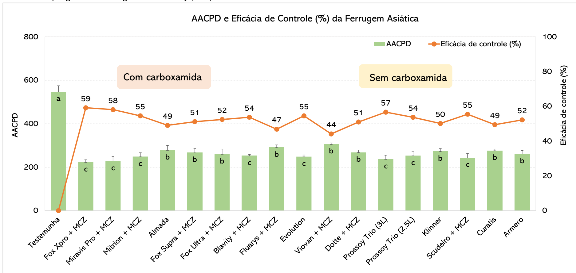
Figura 2. Área Abaixo da Curva de Progresso da Doença (AACPD) e eficácia de controle (%) da ferrugem asiática em plantas de soja submetidas a diferentes programas de fungicidas. Maracaju, MS, 2026.
