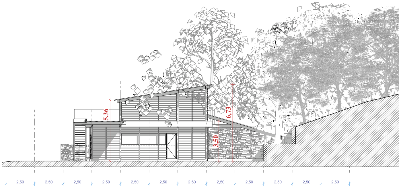
Die Südfassade des zukünftigen Gebäudes
