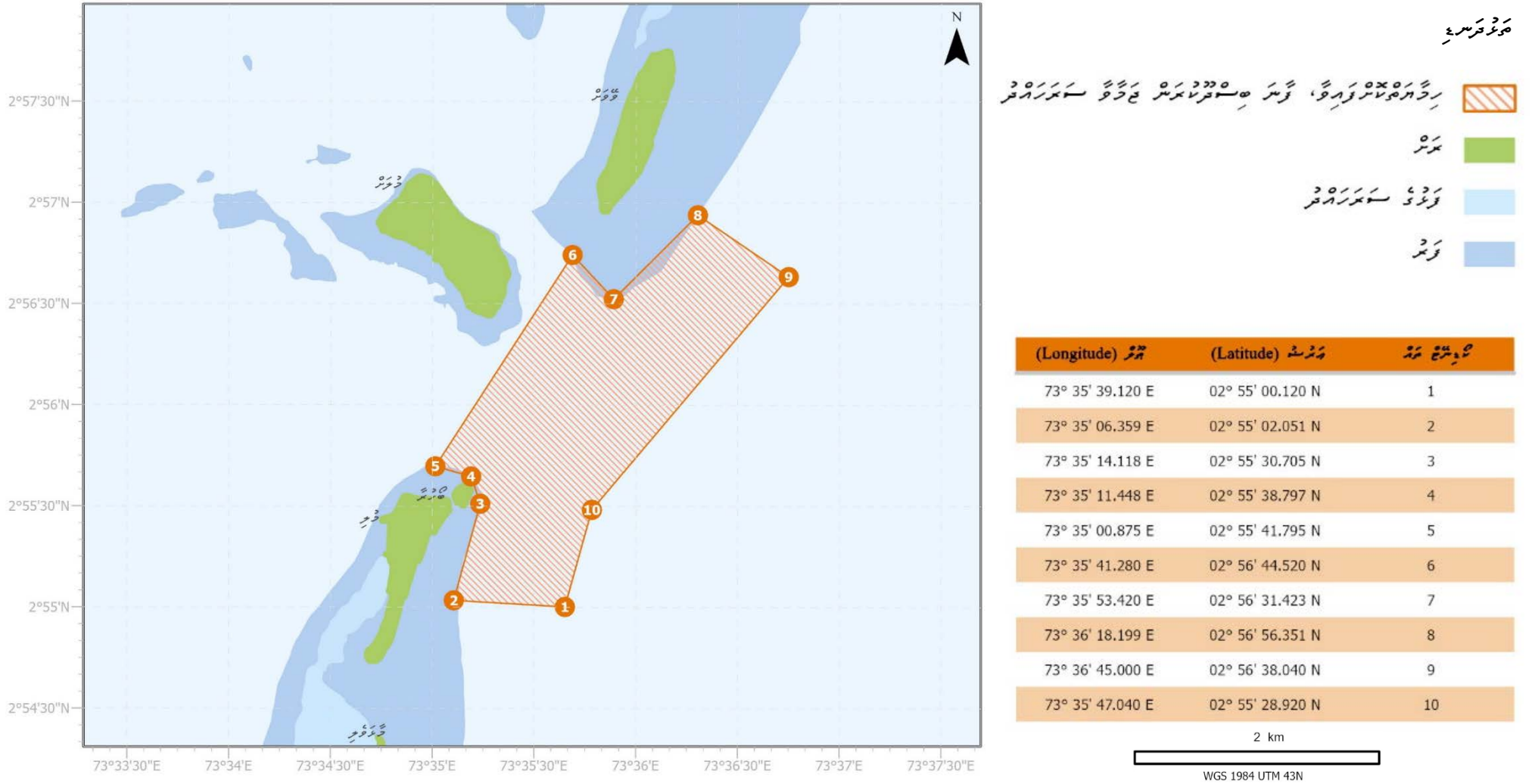
الخطة 4: خطة العمل الخاصة بالمرحلة 2 (د. أ. أ. أ.) - دراسة تقييم الأثر البيئي
