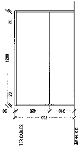
ELEVATION A
