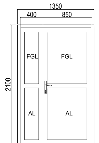
DOOR - A DETAIL
