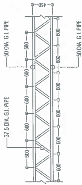
STEEL TRUSS -T1 Scale: 1:50
