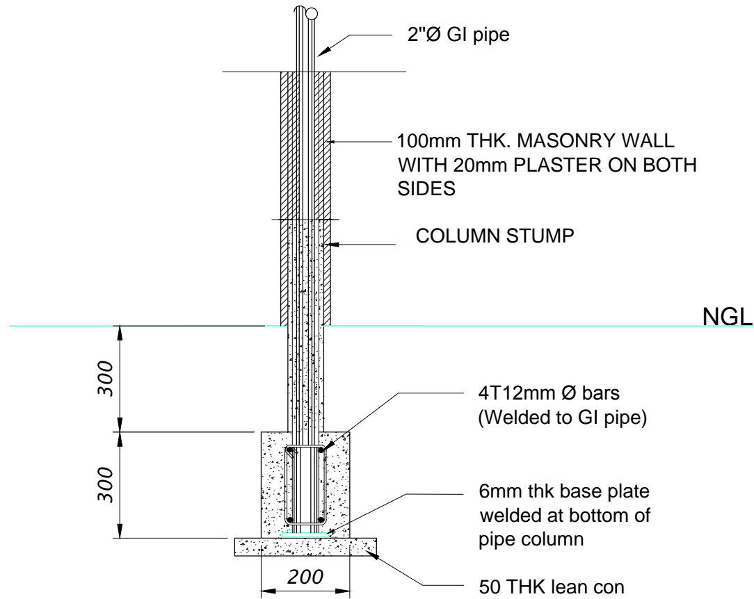
DETAL- COLUMN STUMP
