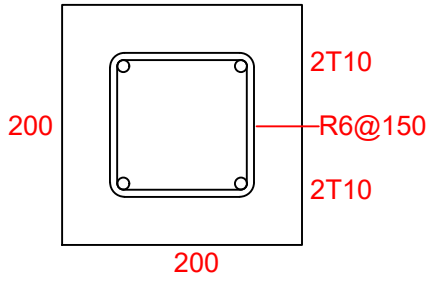
STIFFENER COLUMNS
