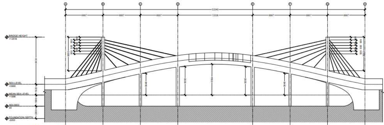
FRONT ELEVATION - E1 1:500
