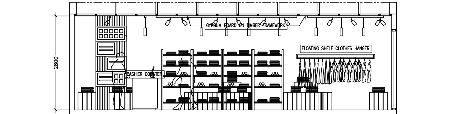
ELEVATION E2-E2
