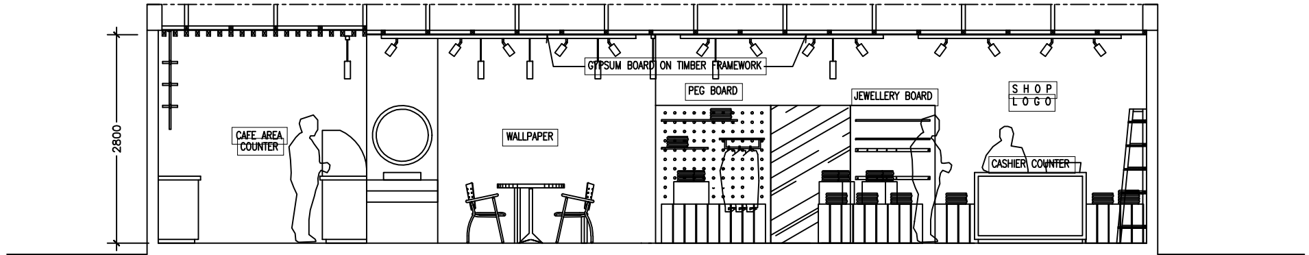
ELEVATION E1-E1
