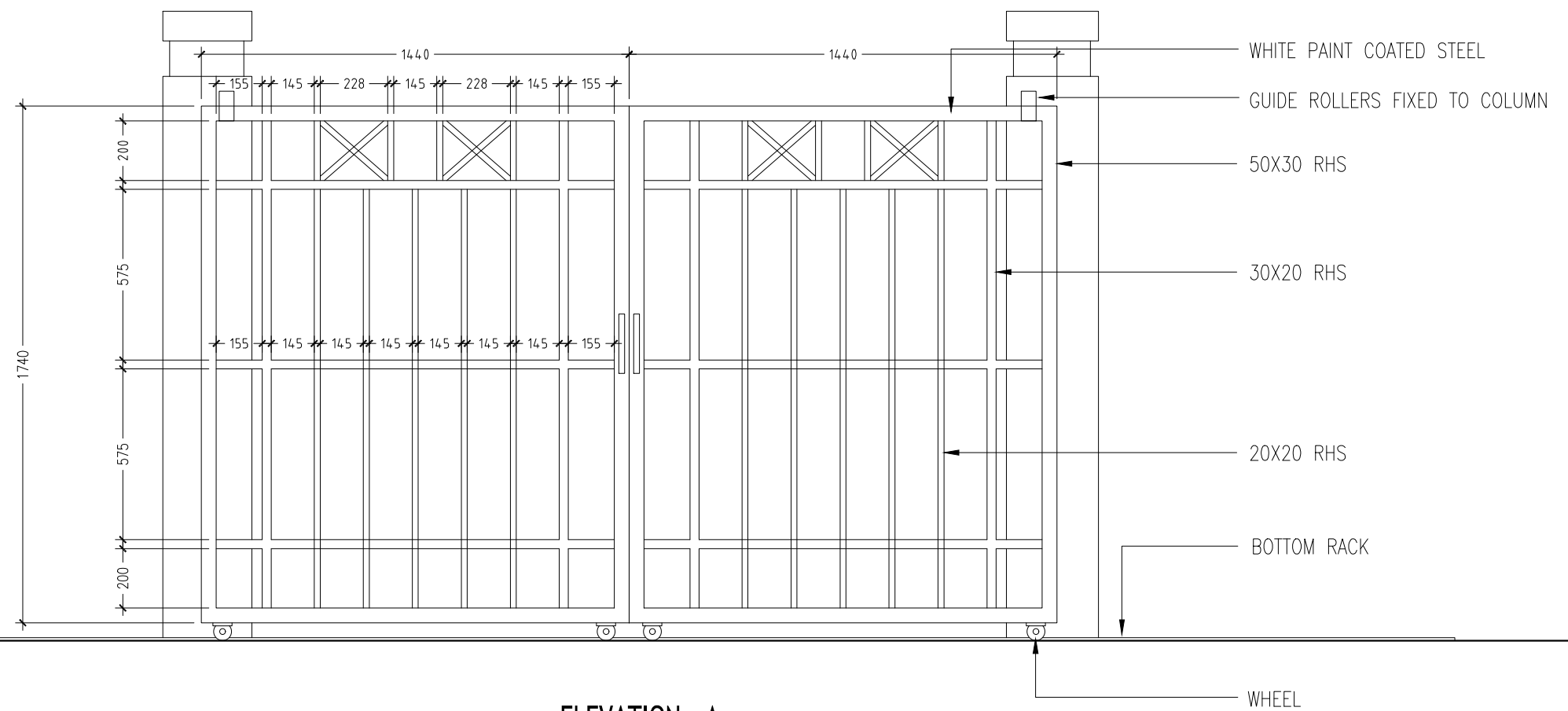
ELEVATION - A
