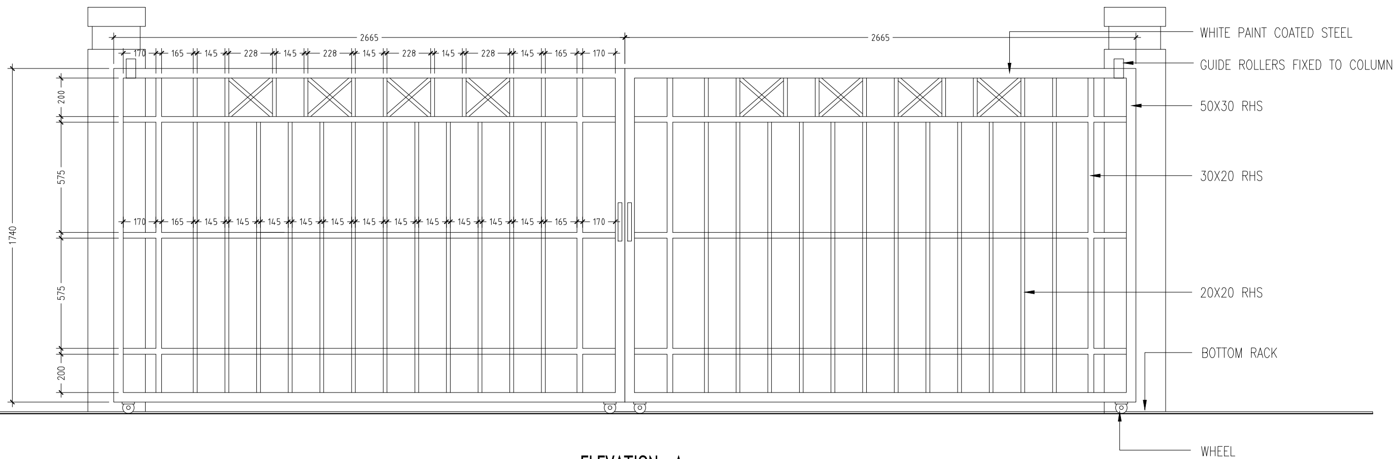
ELEVATION - A
