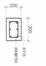
COLUMN C1 1:20
