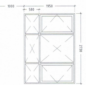
WINDOW W7 1:50
