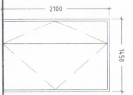
DOOR D5 1:50
