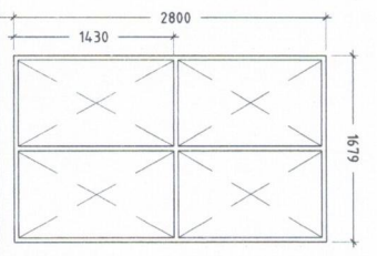
WINDOW W4 1:50
