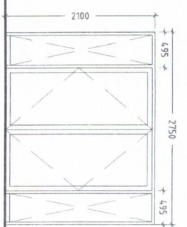
DOOR D7 1:50
