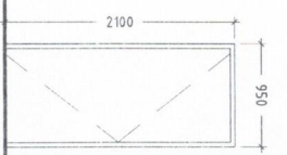
DOOR D4 1:50
