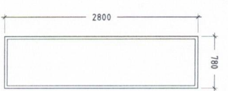
WINDOW W8 1:50
