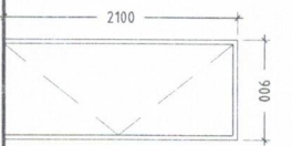
DOOR D2 1:50
