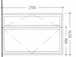
DOOR D6 1:50
