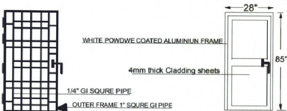
ALUMINIUM DOOR
