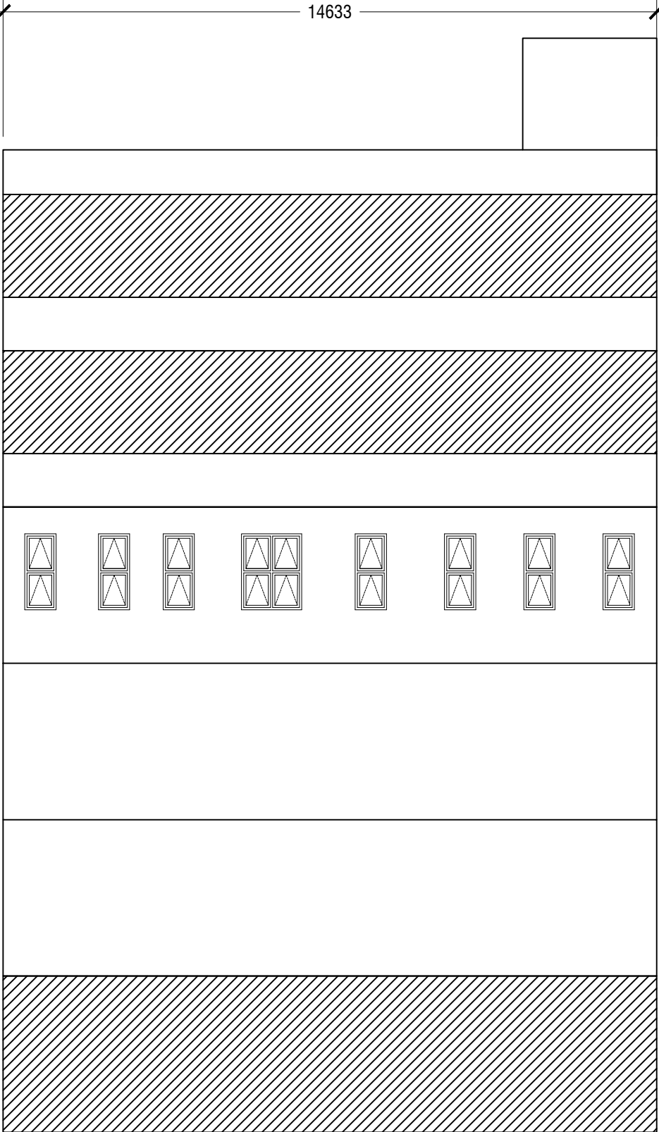
ELEVATION E4
