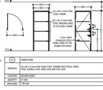
DOOR SCHEDULE SCALE 1:50
