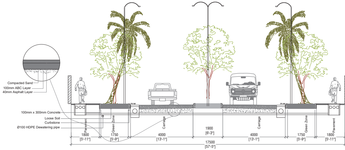
BODUBURU MAGU - SECTION (17.5M)
