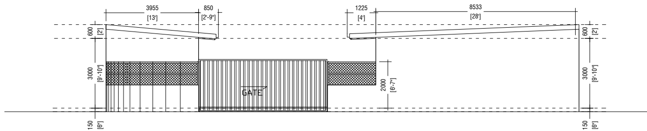
ELEVATION - E2
