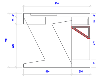
ELEVATION B SCALE: 1:15
