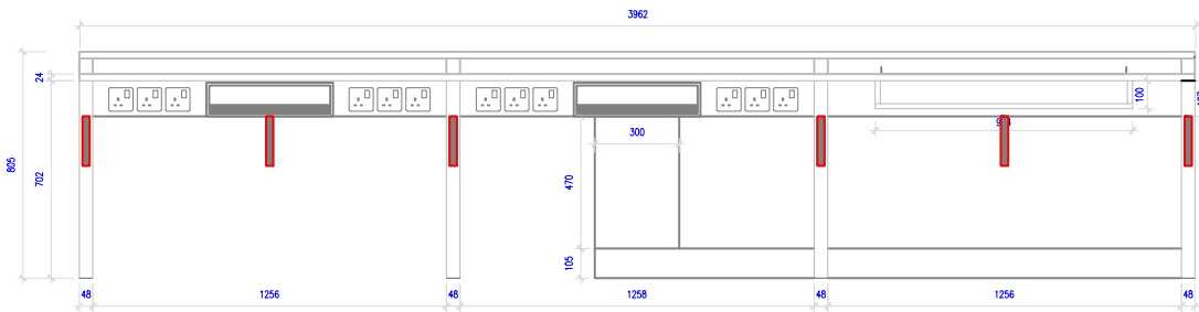
ELEVATION A SCALE: 1:15
