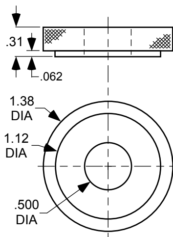
SPACER
