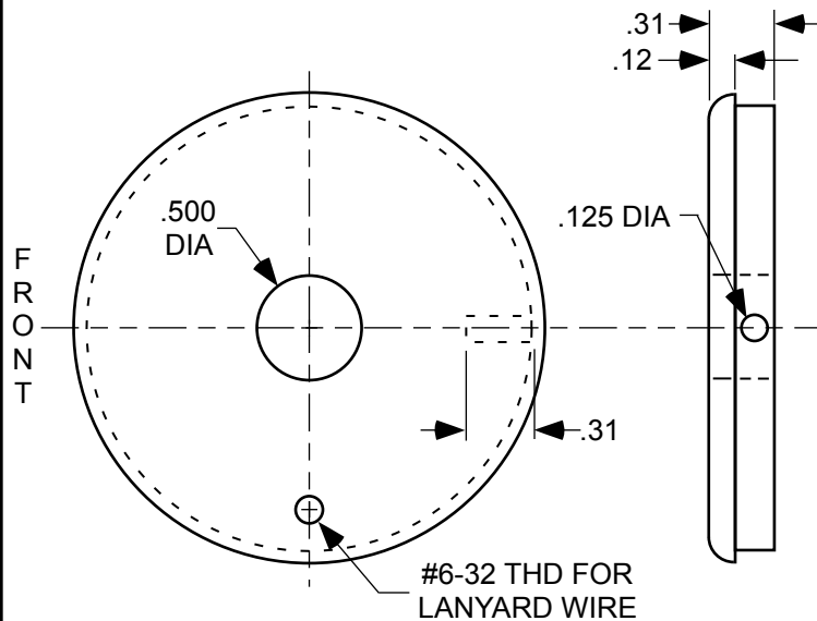
UPPER CAP
