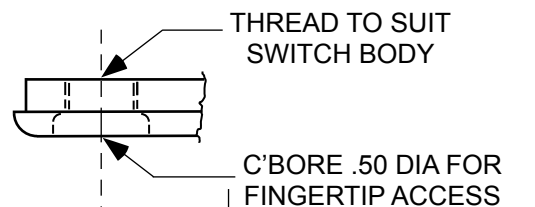
UPPER CAP
