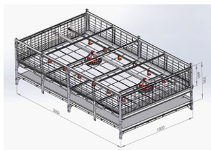
肉鸡笼3000×1800 broiler cage 3000×1800
