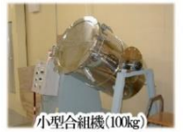
小型合組機(100kg)
