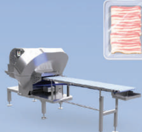
เครื่องสไลด์เนื้ออัตโนมัติ รุ่น NUS-340II อุณหภูมิเนื้อ -2 ถึง 4C
