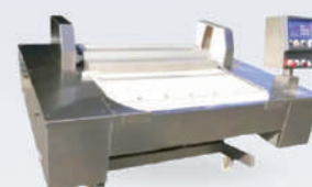
เครื่องแพ็คสุญญากาศ CV-1000 ขนาดแถบซีล 420 มม ปั๊มเยอร์มัน Busch รุ่นสายพานใช้แพ็คแบบต่อเนื่อง
