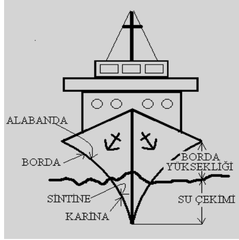
Şekil 1.2: Bir geminin alabanda ve sintinesi
