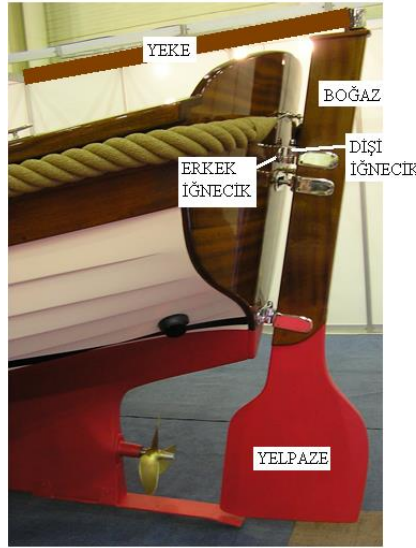
Şekil 1. 3: Dümen
