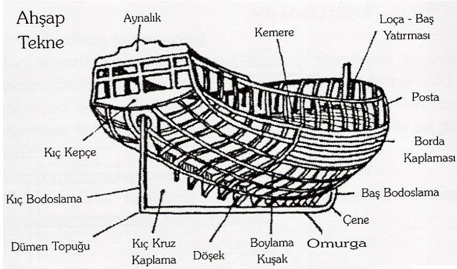
Şekil 1.1: Ahşap tekne yapısı
