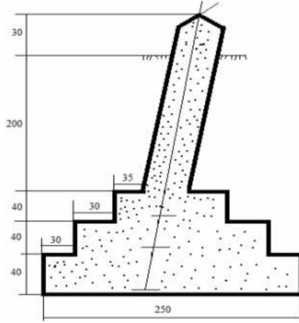
Şekil 2.2: Kademeli temel
