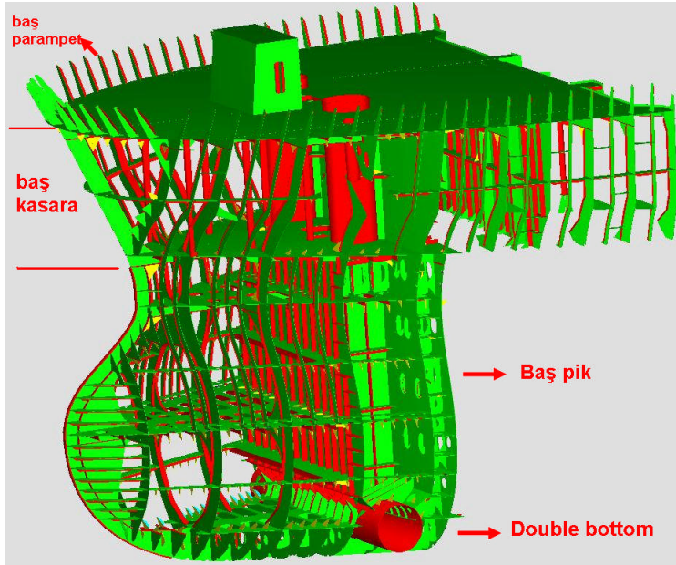
Şekil 1.9: Baş pik, baş kasara, baş parampet
