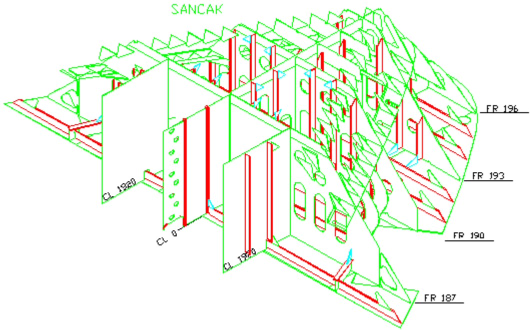
Şekil 1.16: Zincirlik bloęunun ters montaj perspektif resmi
