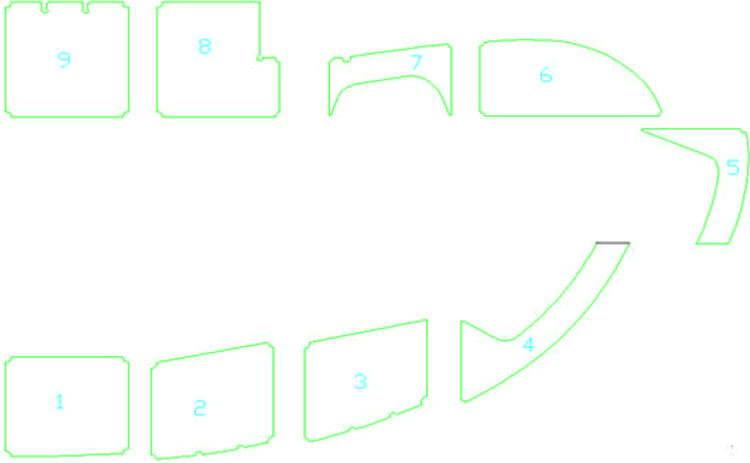
Şekil 2.4:Balb tülani sacları
