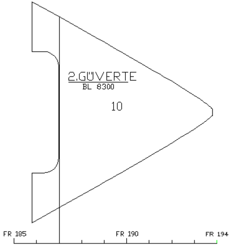
Şekil 2.2: Balb güverte sacı
