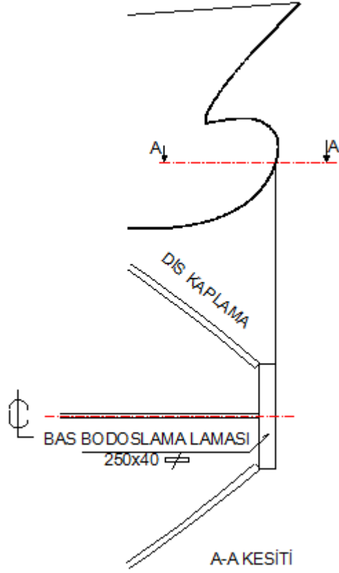
Şekil 1.1: Baş bodoslama formu
