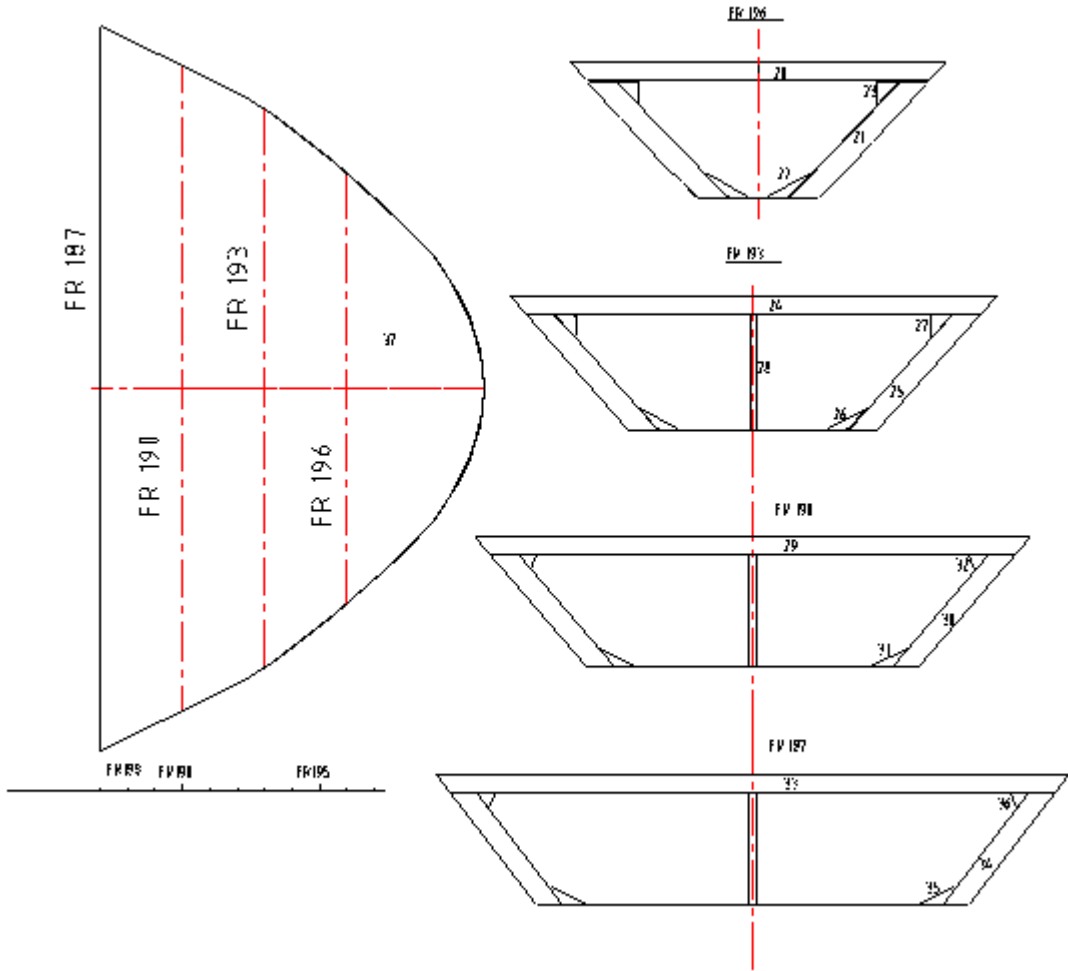
Şekil 1.11: Kasara elemanları
