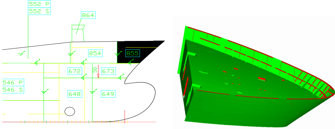
Şekil 1.10: Baş kasara
