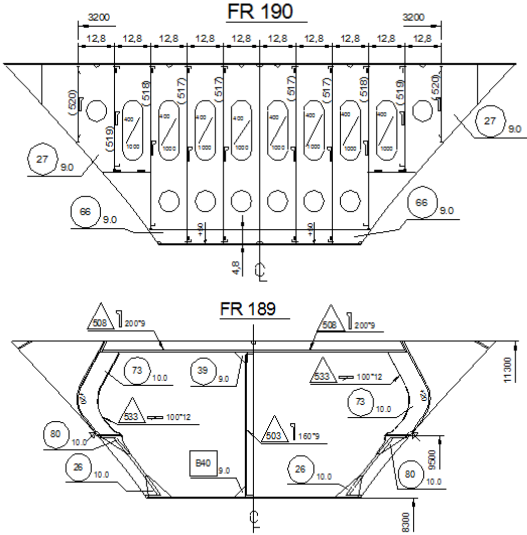
Şekil 1.8: Baş kasara posta kesitleri
