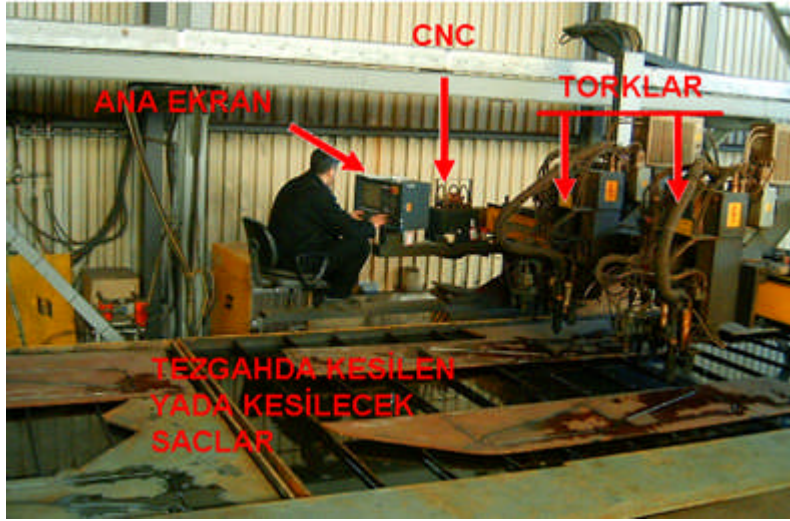
Resim 1.3: CNC tezgâhı
