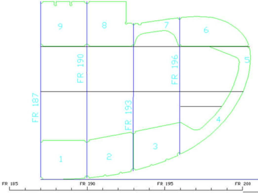
Şekil 2.5: Balb montajı
