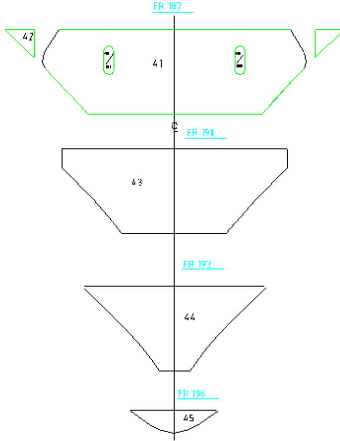
Şekil 1.14: Zincirlik postaları
