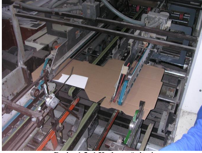
Resim 1.5: 1.Katlama ünitesi
