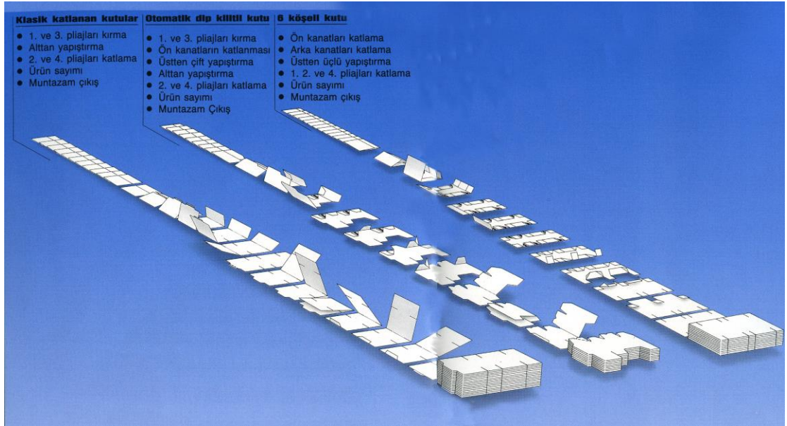
Resim 1.12: Çalışma prensibi
