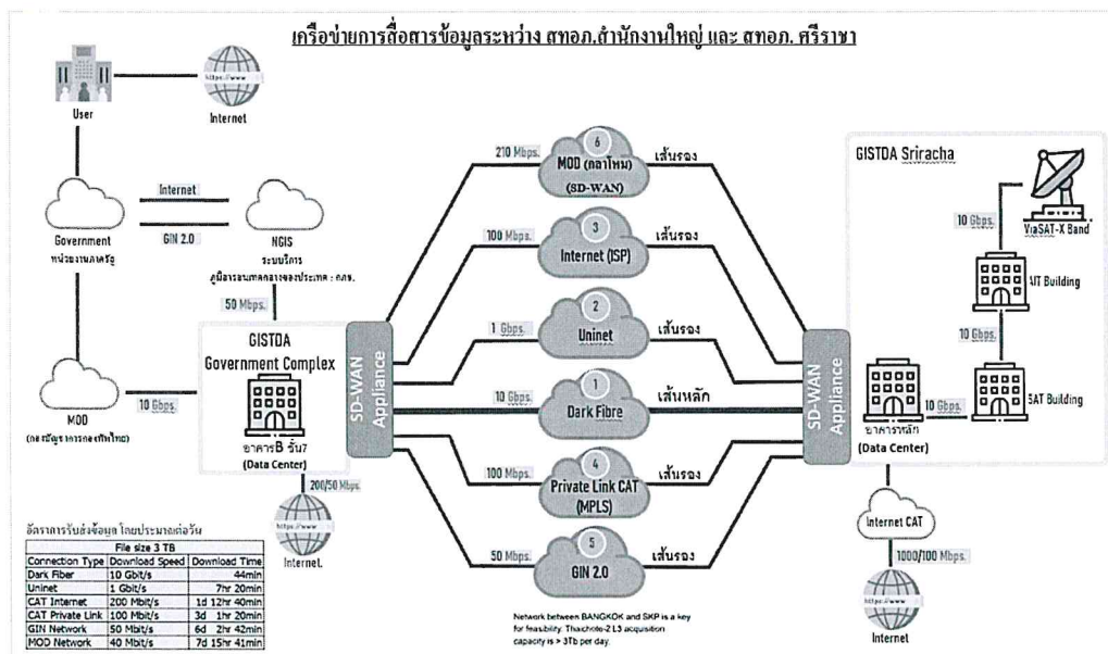
รูปที่ 5 แนวทางการจัดการและรวม WAN Link ระหว่าง สทอ. สำนักงานใหญ่ แจ้งวัฒนะ กับ สทอ. ศรีราชา
