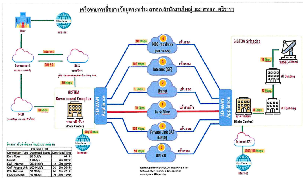
รูปที่ 5 แนวทางการจัดการและรวม WAN Link ระหว่าง สทอภ. สำนักงานใหญ่ แจ้งวัฒนะ กับ สทอภ. ศรีราชา
