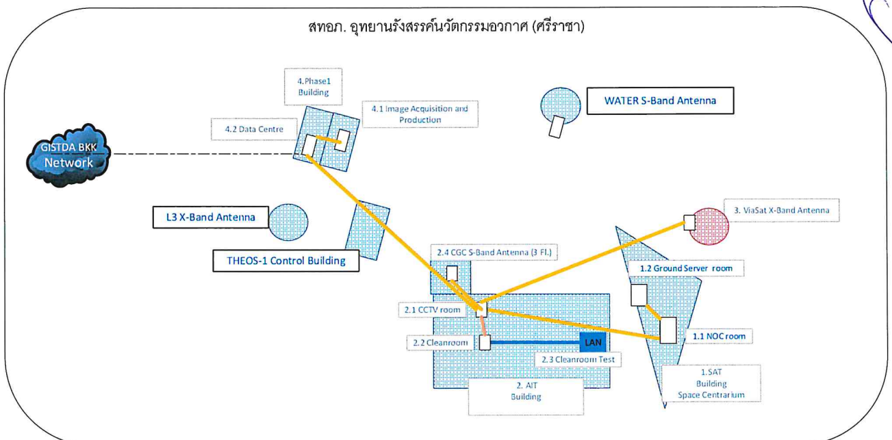
รูปที่ 2 งานติดตั้งสายใยแก้วนำแสง (Fiber Optic) ระหว่างอาคารและภายในอาคาร ของ สทอภ. อุทยานรังสรรค์นวัตกรรมอวกาศศรีราชา
