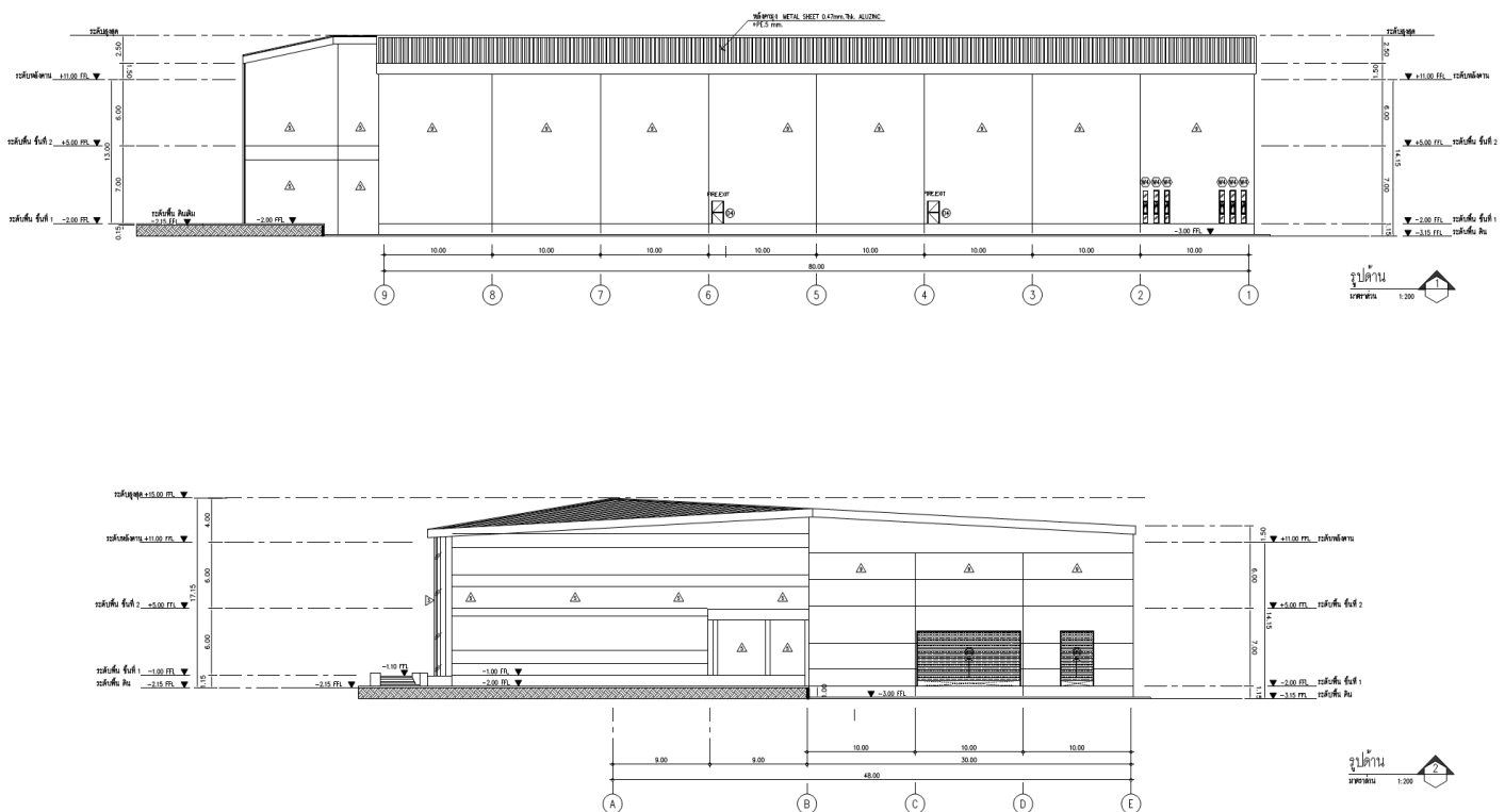
ภาพที่ 2 ภาพตัดขวางอาคาร ห้อง Clean Room
