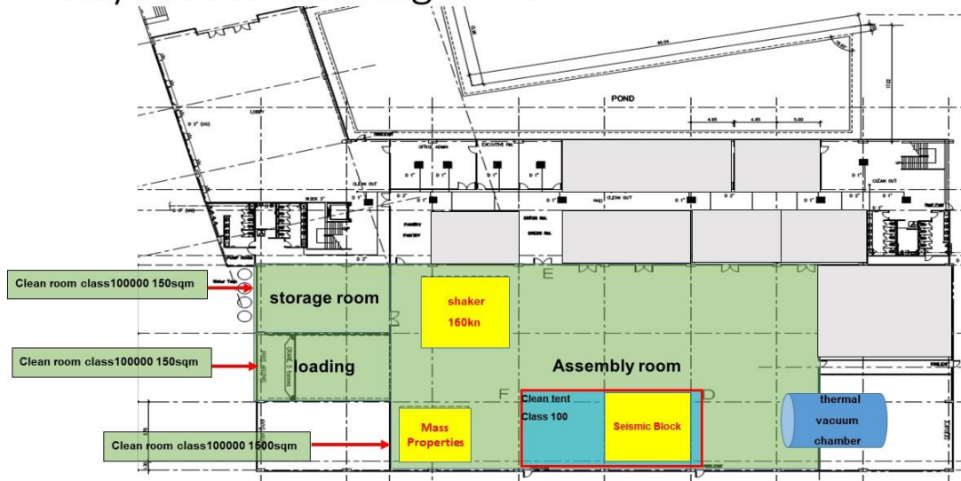
ภาพ Equipment Installation plan
