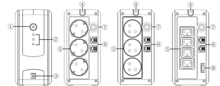
UT700EIG / UT850EG / UT850EIG (Schuko/French/IEC Outlet)
