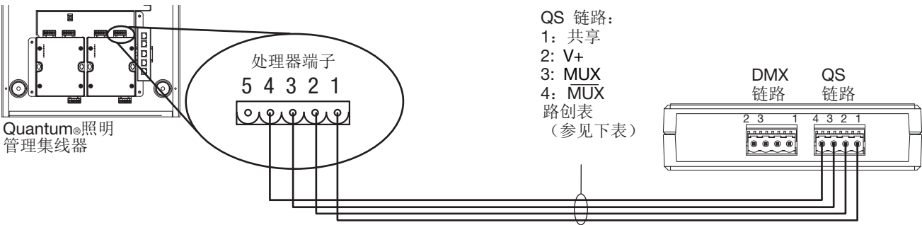
QS链路接线尺寸（检查与您所在区域的兼容性）
