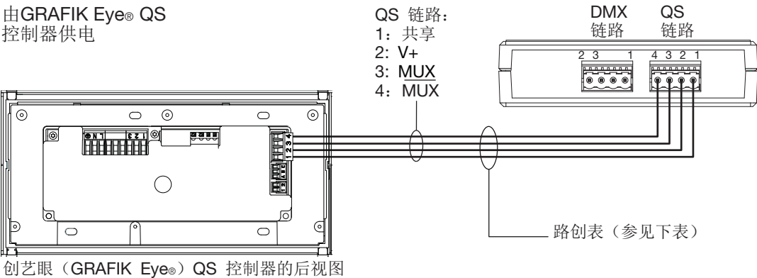
由 QS 链路电源供电 注：GRAFIK Eye® 控制器上的端子2不连接至 QS 链路电源。
