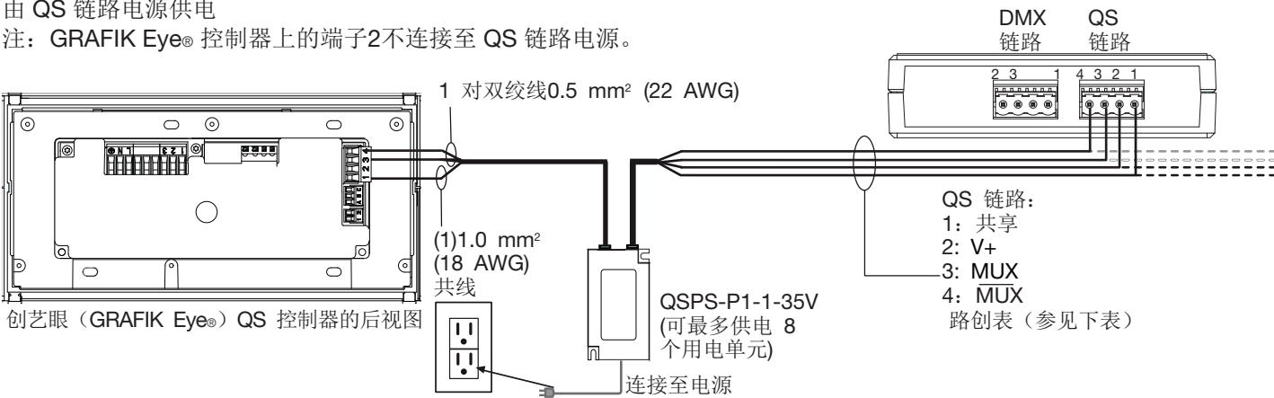
由Quantum®照明管理集线器供电
