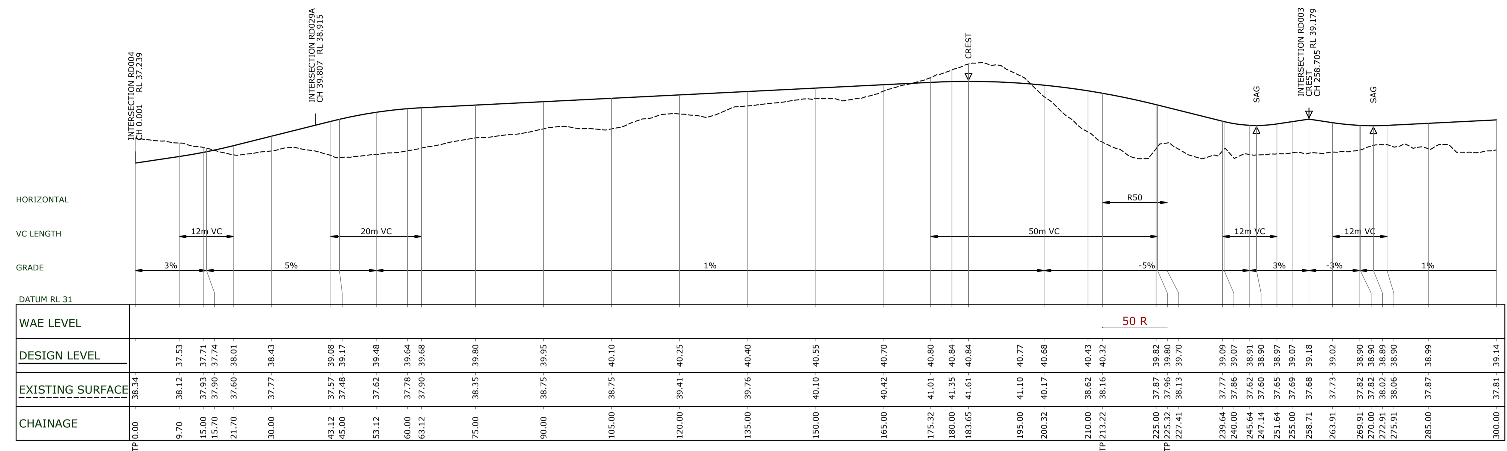
RD029 LONGITUDINAL SECTION 1:500 HORI. 1:100 VERT.
