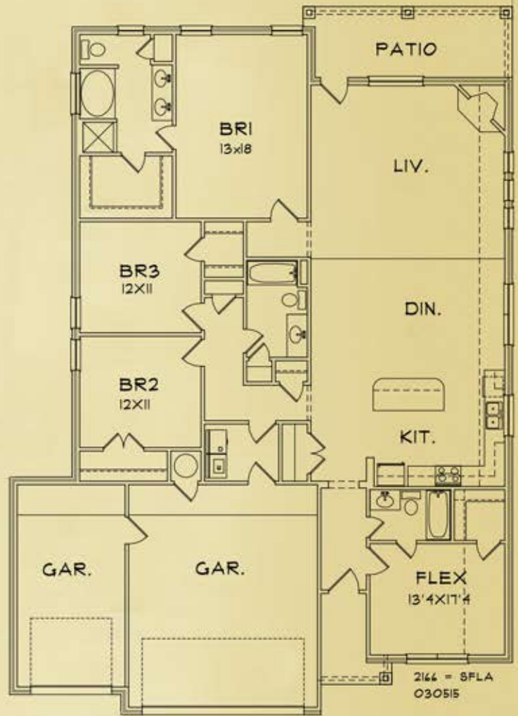
EF 2166 2014 PLAN
