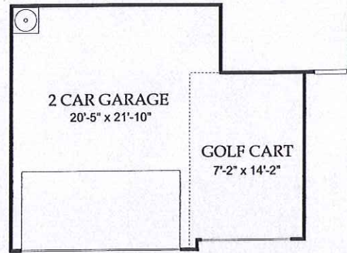
Optional Golf Cart Garage
