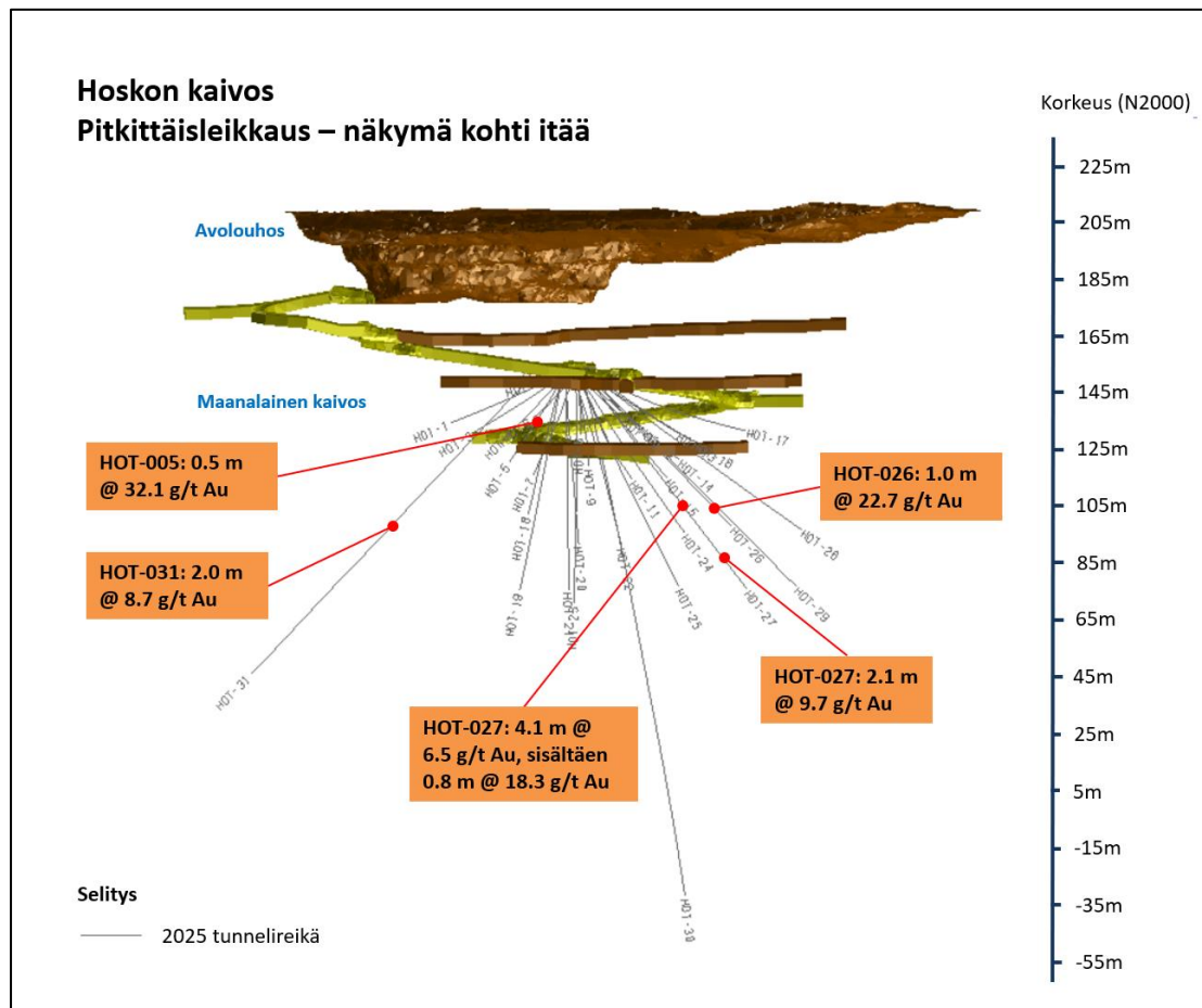
Kuva 1 – Hoskon kaivoksen uusien kairareikien sijainnit pitkittäisleikkauksessa
