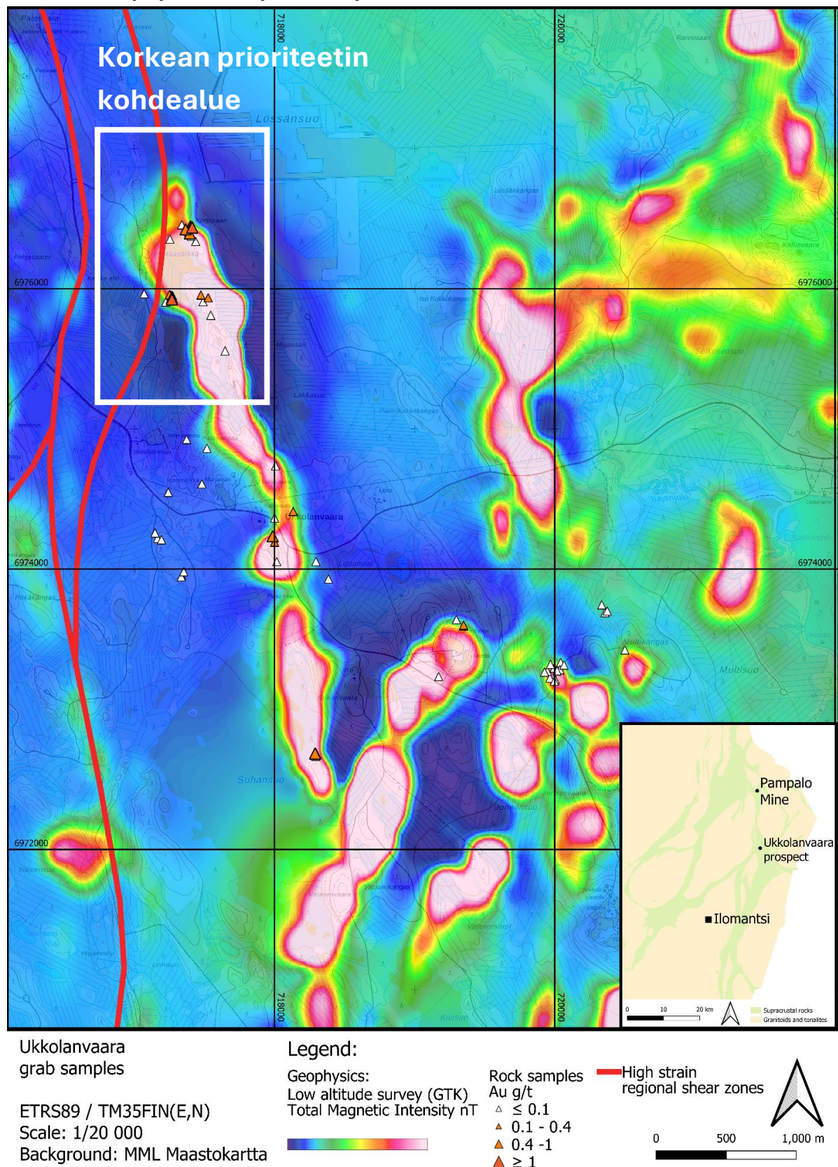
Kuva 1 – Ukkolanvaaran 2024 kallioperäkartoitusohjelman näytteiden sijaintikartta, Pohjana magneettinen totaali-intensiteettikartta, joka havainnollistaa vahvasti magneettisen Ukkolanvaaran rautamuodostuman.
