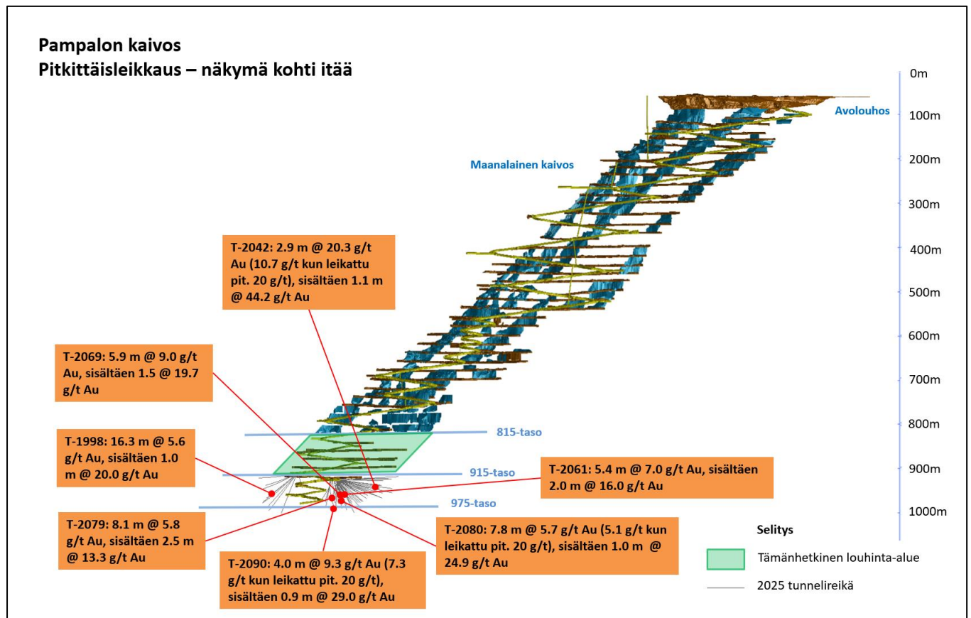
Kuva 1 – Pampalon kaivoksen uusien kairareikien sijainnit pitkittäisleikkauksessa
