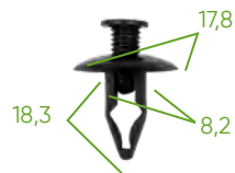
13063 ASSORTIMENTO CLIP DI FISSAGGIO 6 PCS P/52891
