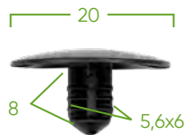
13065 ASSORTIMENTO CLIP DI FISSAGGIO 15 PCS P/52891
