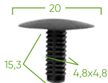
13089 10X KUNSTSTOFF-CLIPS FÜR NISSAN (IN SET REF. 52894)
