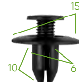
13088 10X KUNSTSTOFF-CLIPS FÜR NISSAN (IN SET REF. 52894)
