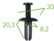
13098 ASSORTIMENTO CLIP DI FISSAGGIO 4 PCS P/52895
