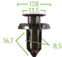
13102 ASSORTIMENTO CLIP DI FISSAGGIO 5 PCS P/52895
