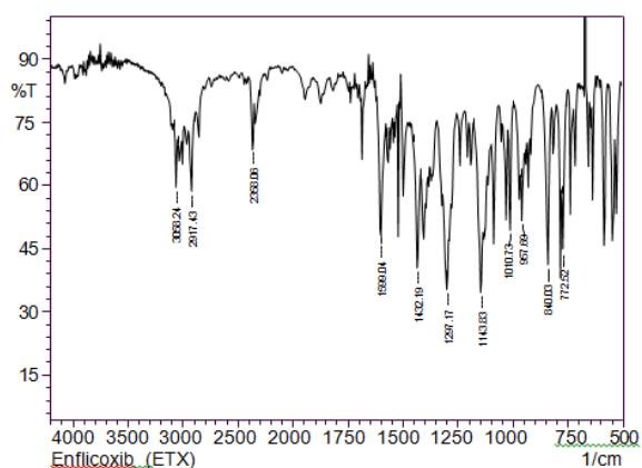
Fig. 6: IR spectrum of Enflucixib.
