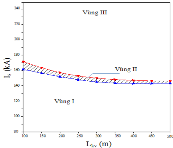
Hình 8. Phân bố các vùng xảy ra phóng điện trên các pha không treo CSV khi thay đổi khoảng vượt, R_{td2} = 10\Omega , R_{td3} = 5\Omega
