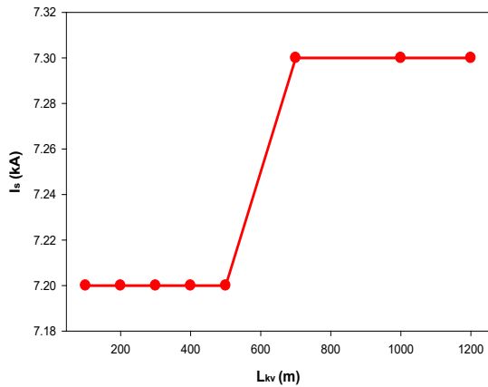
Hình 14. Quan hệ giữa dòng điện gây phóng điện cột 3 theo chiều dài khoảng vượt khi sét đánh vào dây pha, R_{td2}=10\Omega , R_{td3}=5\Omega
