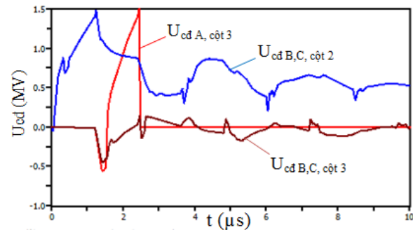
Hình 6. Điện áp trên cách điện cột 2 và cột 3 khi CSV pha A của cột 2 làm việc, phóng điện xảy ra trên cách điện cột 3
