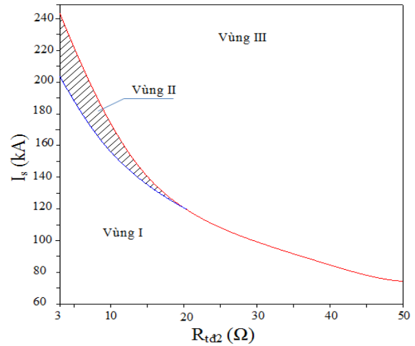
Hình 9. Phân bố các vùng xảy ra phóng điện trên cách điện khi sét đánh vào cột 2, CSV cột 2 làm việc, khi R_{td3} = 5\Omega .
