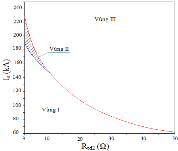
Hình 7. Phân bố các vùng xảy ra phóng điện trên cách điện khi sét đánh vào cột 2, CSV cột 2 làm việc, khi R_{td3} = 5\Omega . Vùng I: không phóng điện, vùng II: phóng điện trên cách điện cột 3, vùng III: phóng điện trên cách điện cột 2
