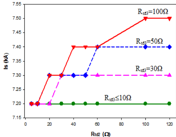
Hình 13. Quan hệ giữa dòng điện gây phóng điện cột 3 khi sét đánh dây pha A với R_{td3} thay đổi từ 10Ω đến 100Ω
