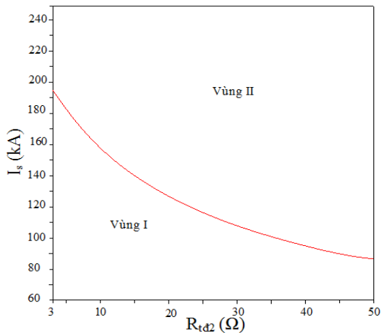
Hình 11. Phân bố các vùng xảy ra phóng điện trên cách điện khi sét đánh vào cột 2, CSV cột 2 làm việc, khi R_{td3}=5\Omega .
