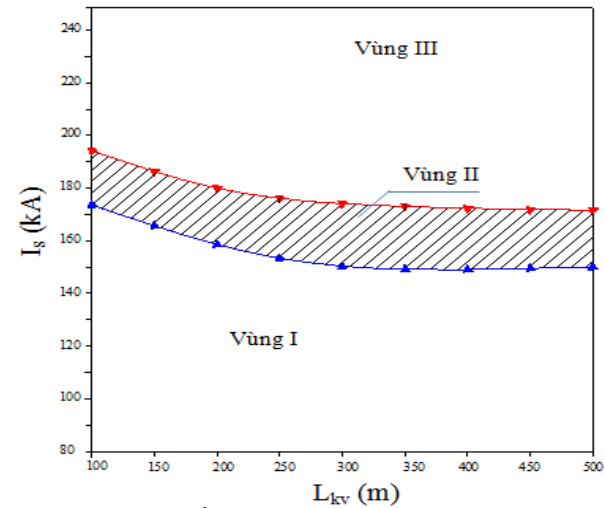
Hình 10. Phân bố các vùng xảy ra phóng điện trên các pha không treo CSV khi thay đổi khoảng vượt, R_{td2} = 10\Omega , R_{td3} = 5\Omega
