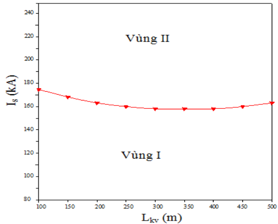
Hình 12. Phân bố các vùng xảy ra phóng điện trên các pha không treo CSV khi thay đổi khoảng vượt, R_{td2}=10\Omega, R_{td3}=5\Omega
