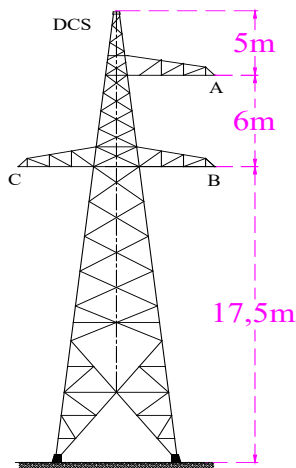
Hình 5. Kích thước cột 220kV loại Đ212A
